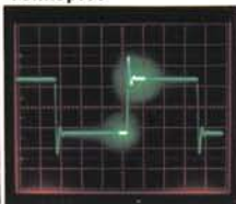
Rechteckverhalten eines konventionellen Tonkopfes
